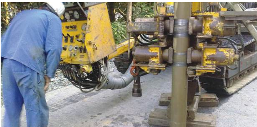
Bohrgerät der GKB bei der Sondier-Bohrung
